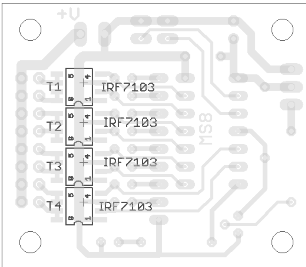
Abb.1 Bestückungsplan Leiterbahnseite, Aufsicht auf die Lötseite
